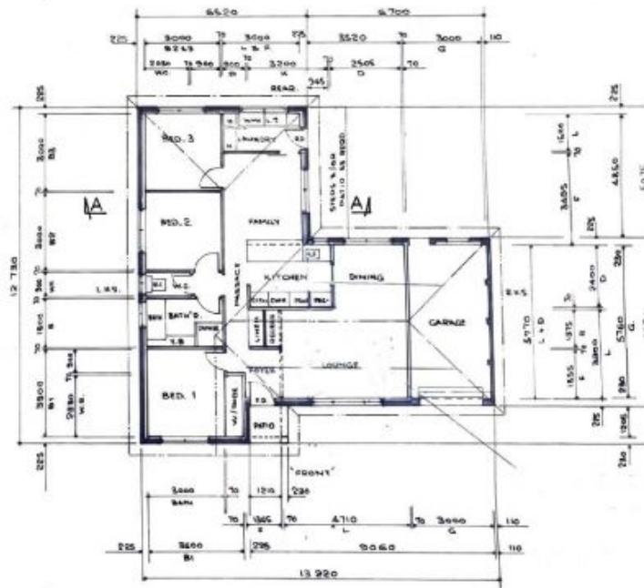
FLOOR PLAN 1 : 100
