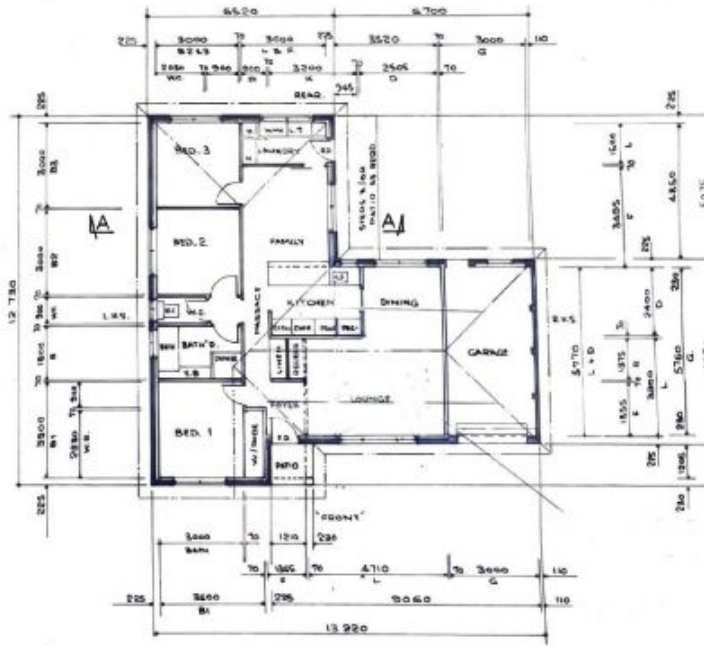
FLOOR PLAN 1 : 100
